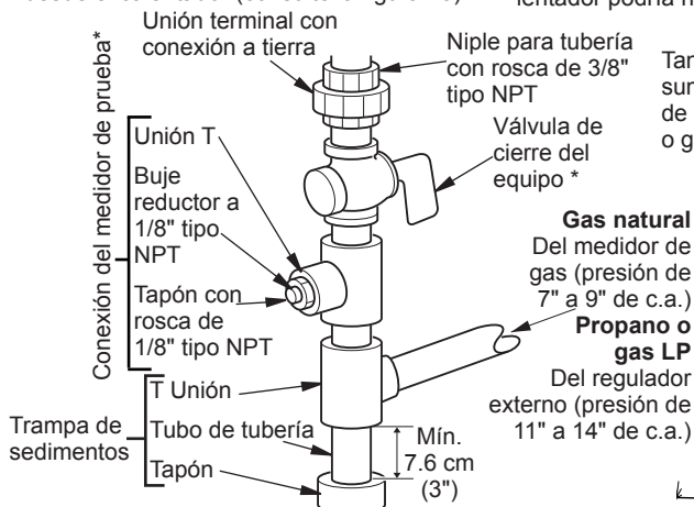
Figura 15 - Conexión de gas
