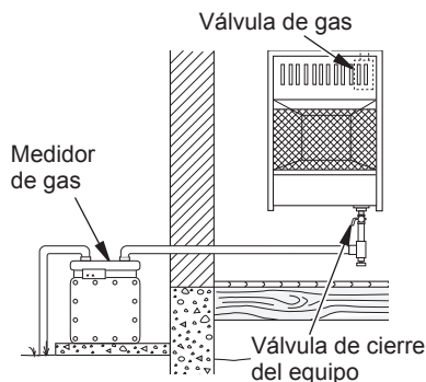
Figura 18 - Suministro de gas natural
